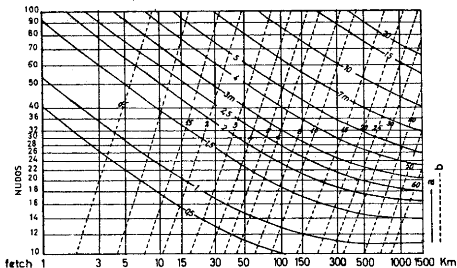
Fig. 2.—Oleaje calculado en función de la velocidad del viento, duración del mismo y fetch (según BRETSCHNEIDER, 1952; adaptado). a = altura significativa en metros; b = duración mínima del viento en horas.
